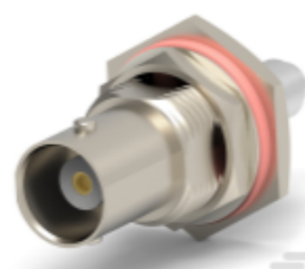
TE 系列/零件编号 5413771-3 JACK BLKHD, COMML BNC, HEX CRIMP
