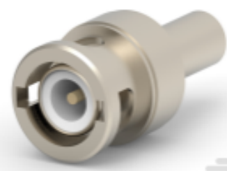
TE 系列/零件编号 5-1634500-2 BNC Str Plg Hex 50Ohm Nickel Pltd RG58C/
