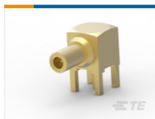
TE 系列/零件编号 1-1337481-0 SMB R/A PCB Skt 50Ohm Gold Plt
