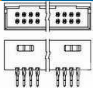
TE 系列/零件编号5-103337- 6 16 MODII HDR DRST SHRD A/PIN
