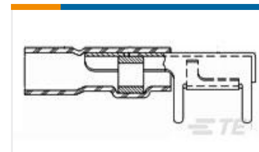
TE 系列/零件编号 601072-000 D-607-10
