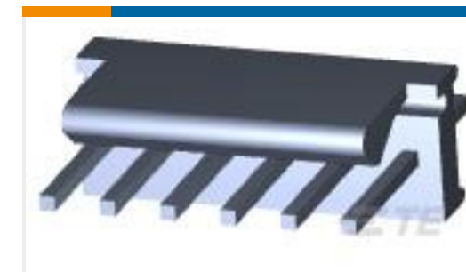
TE 系列/零件编号3-641126- 6 06P MTA100 HDR ASY FL /STR LF
