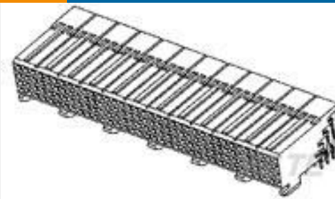
TE 系列/零件编号147055-1 11/12 MODII 2PC CE RCPT ASSY
