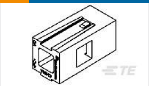
TE 系列/零件编号1445729-2 MTG BRKT RND HOLE
