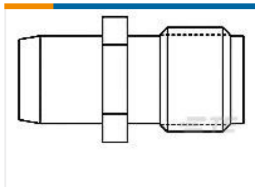
TE 系列/零件编号1059716-1 4582 2240 02
