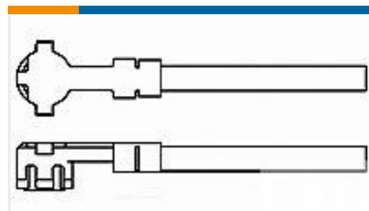
TE 系列/零件编号1064542-1 9960 2510 24
