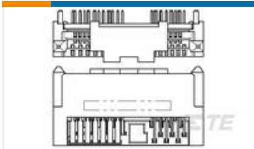
TE 零件编号2129116-3 SLIMLINE SATA PLUS REC CL5.6H, AU G/F
