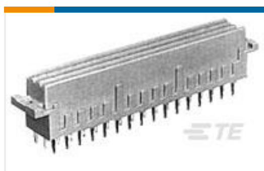
TE 零件编号100108-4 32P.IEC-F FEM.CONN.
