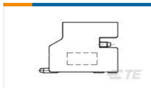
TE 零件编号1775469-2 HPI CONN., 2.0MM, R/A, SMT, 2P, 80U"
